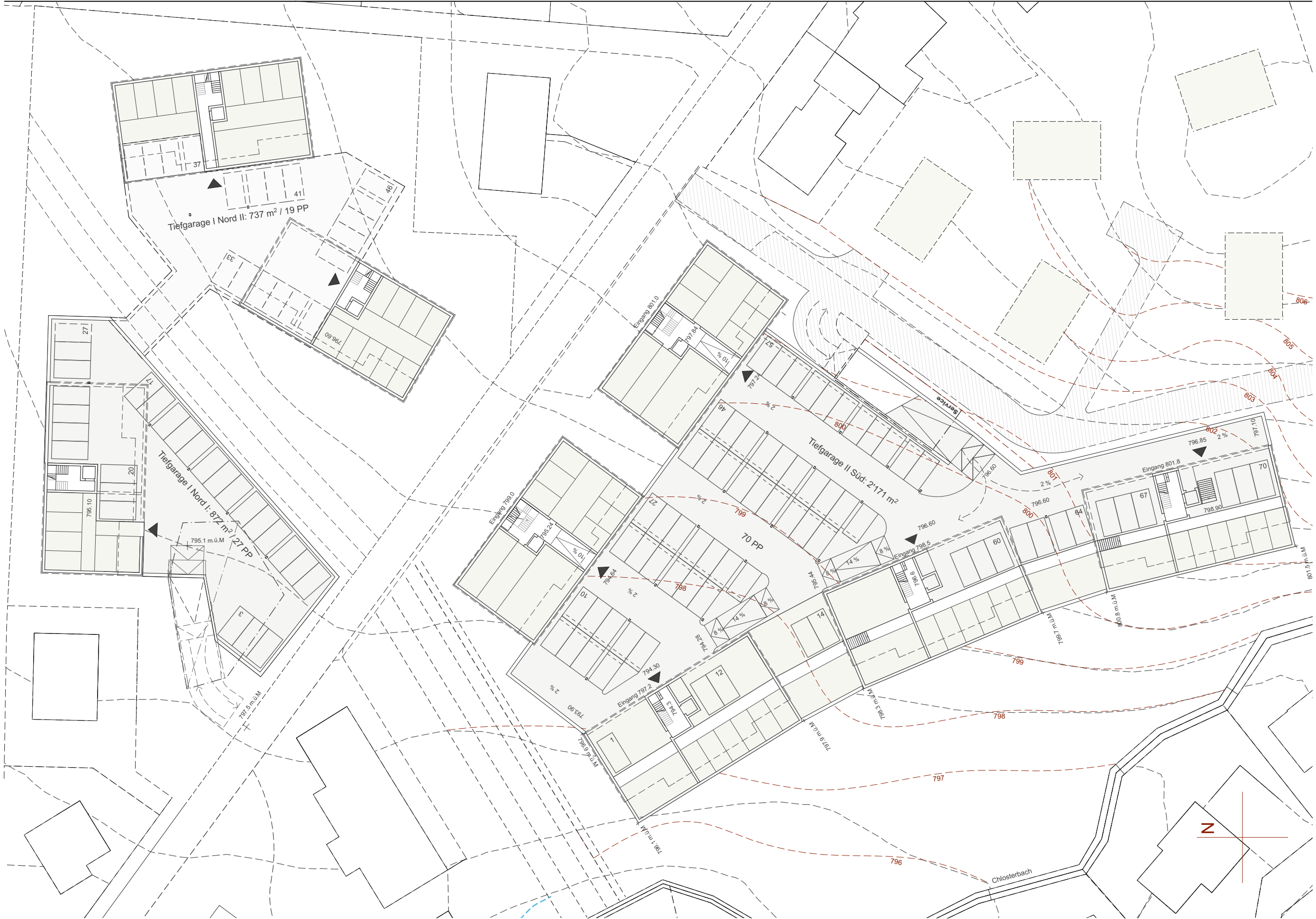
Untergeschossplan 1:500
