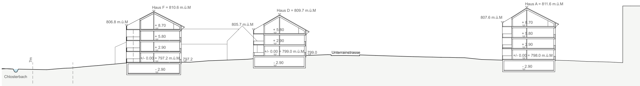
Schnitt A-A
