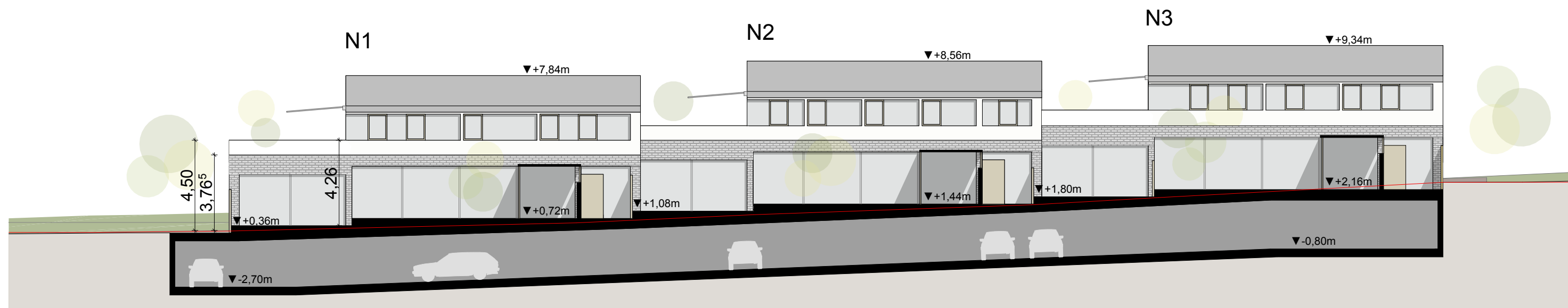
Häuser Nord - Ansicht Süd + Schnitt Tiefgarage M 1:200
