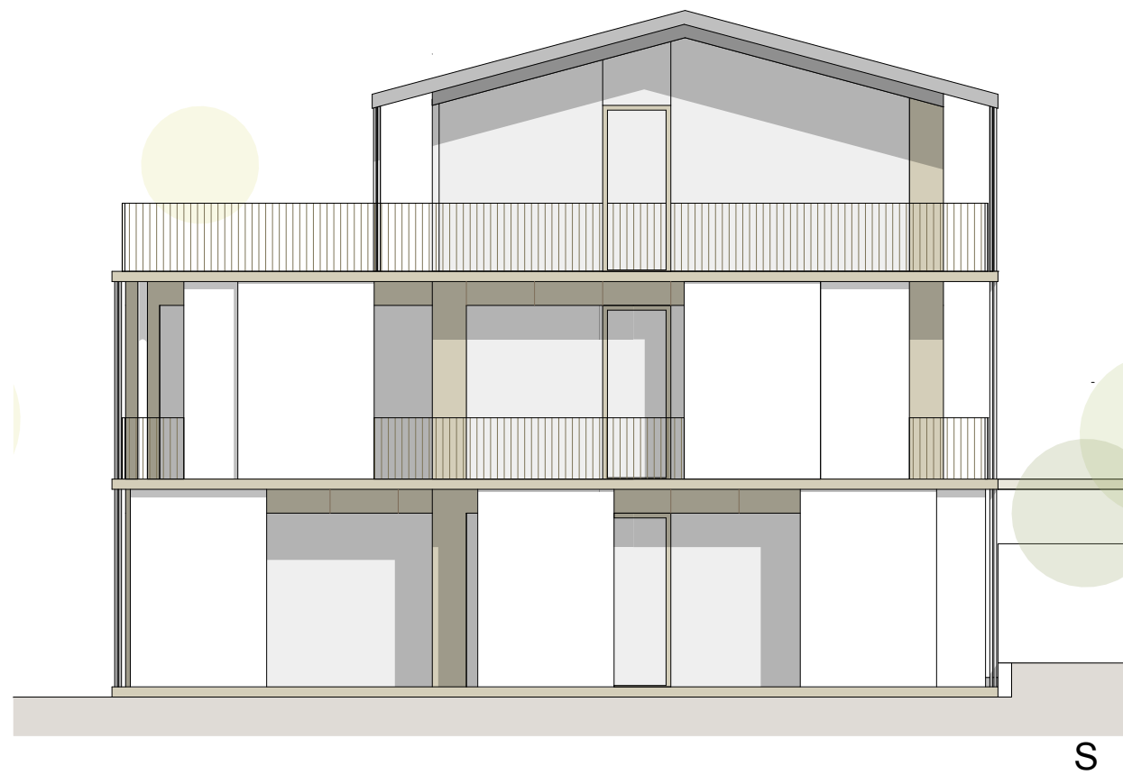
Ansichten Häuser Süd M 1:100
