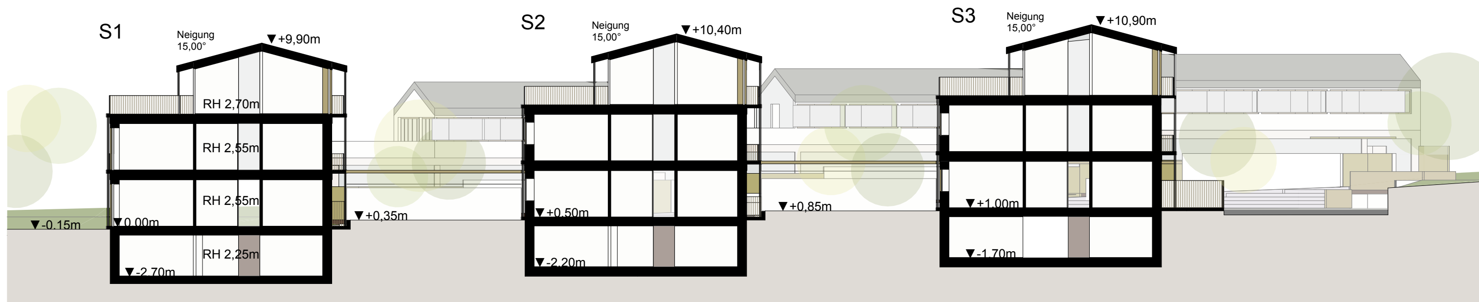
Häuser Süd - Schnitt W-O M 1:200
