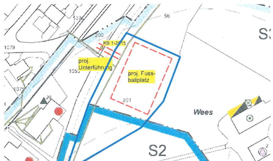
Abb. 6 Übersichtsplan mit Bauprojekt und Kernbohrung KB 1-2015 (o. M.)
